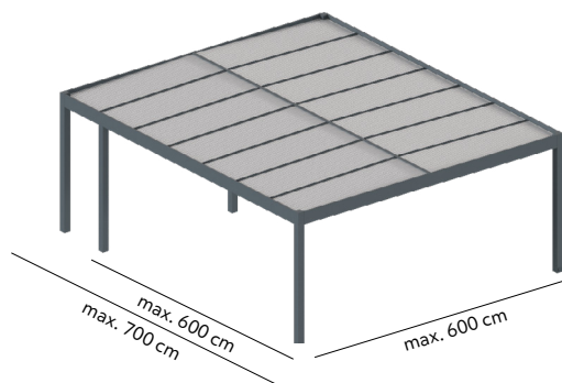
Dach dwupołaciowy | Double-pitched roof
