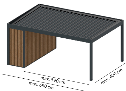
Carport jednostanowiskowy | One-station Carport
