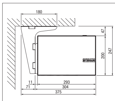
Montaż stropowy
